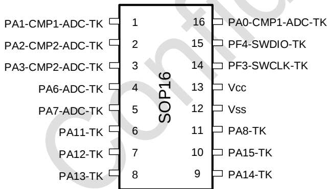
图 3-11 SOP16 Pinout2 PY32T020W2xS7-B (Top view)
